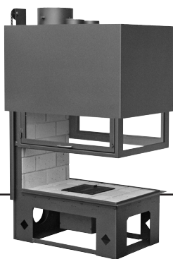
vue perspective
