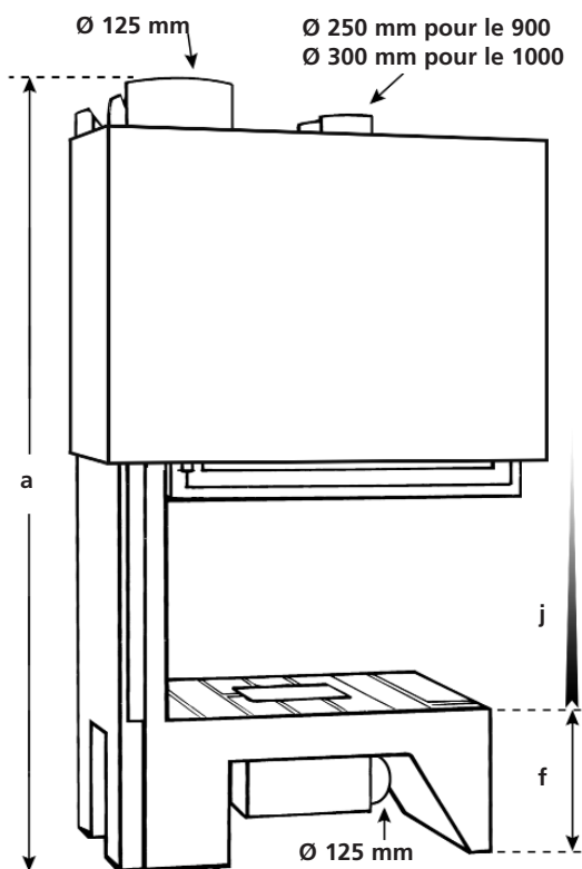
vue perspective
